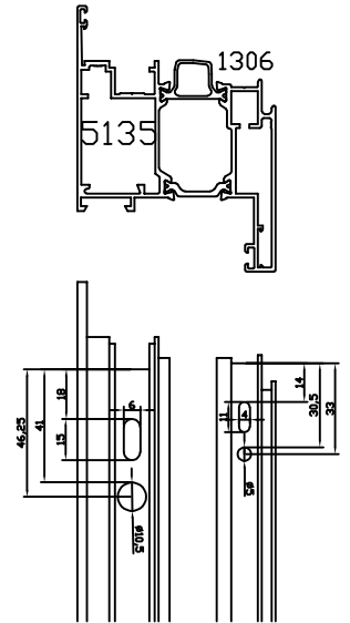
HOJA BALCONERA
