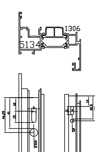
HOJA VENTANA
