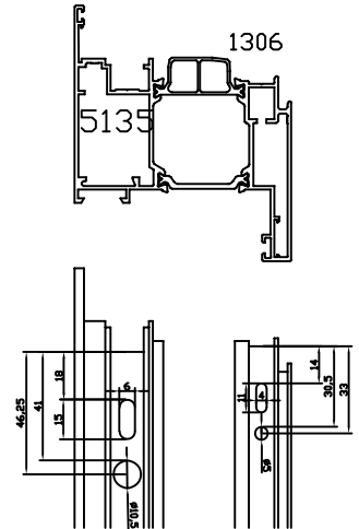
HOJA BALCONERA
