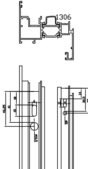
HOJA VENTANA
