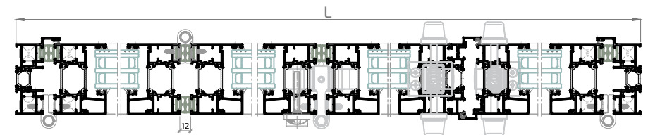
Sección A-A'
