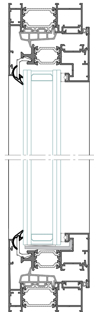
Sección B-B'
