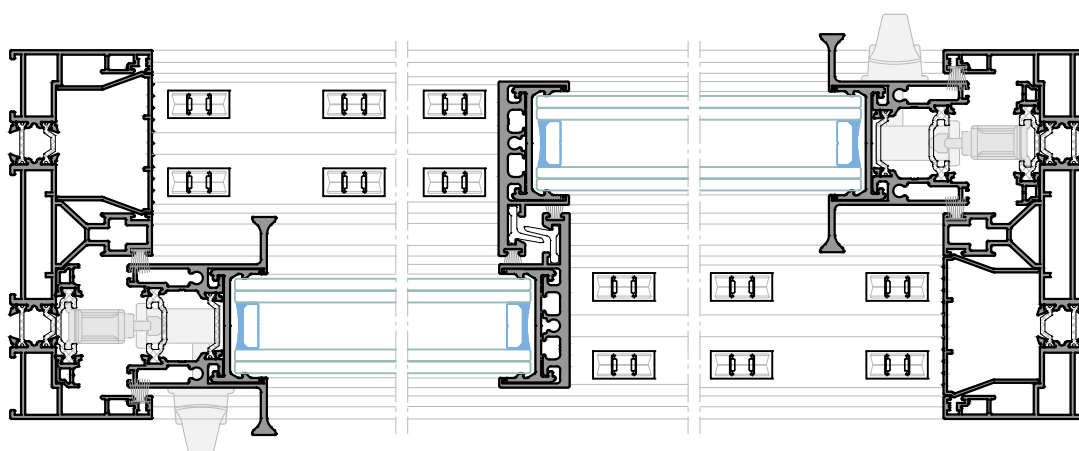
Sección A-A'
