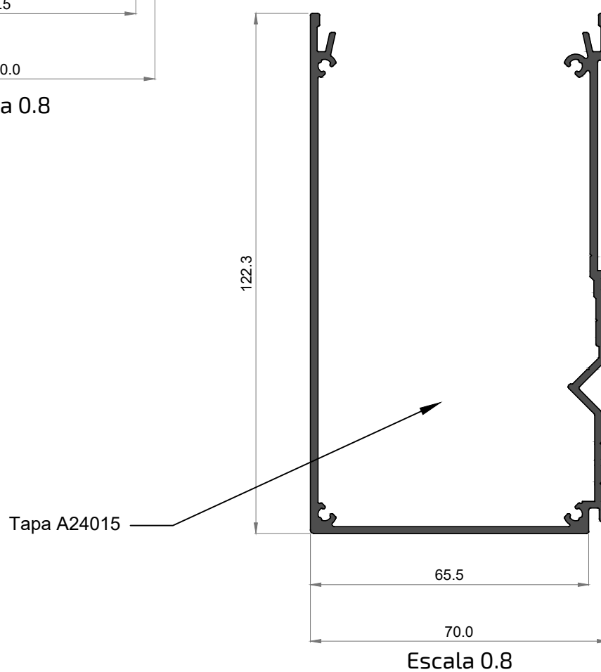
20977 Canalón 100 IBIZA I-LINE
