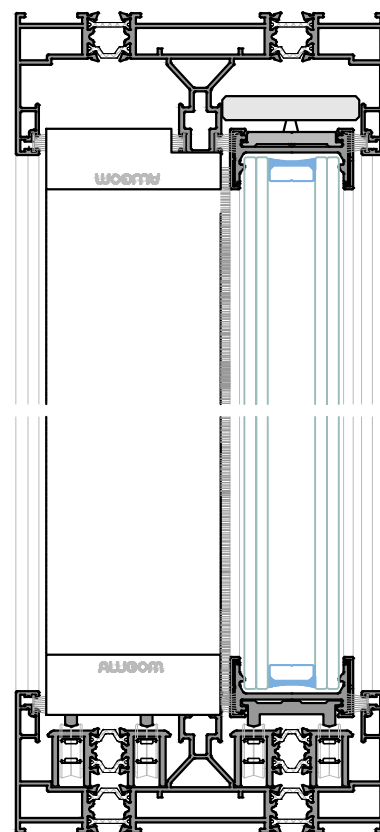
Sección B-B'
