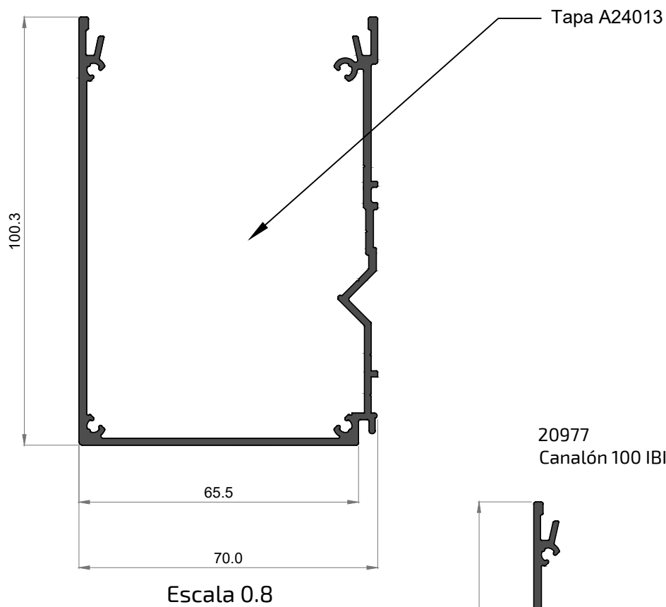
20979 Canalón 100 IBIZA
