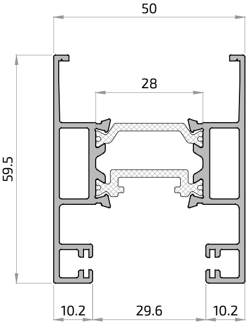
21244L Hoja lateral cierre Matra NG
