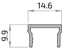
21209 Tapa clip
