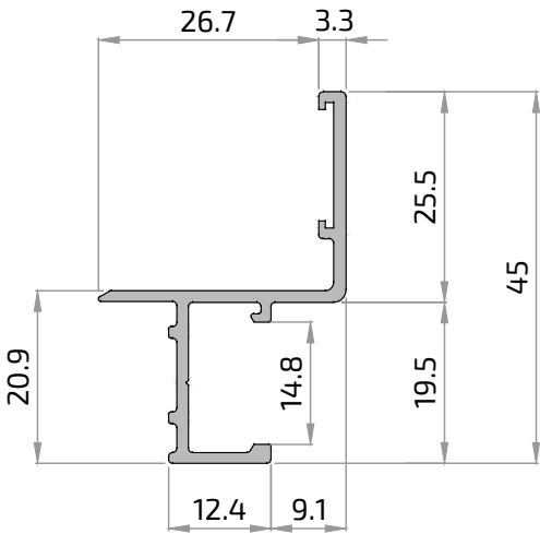
21251 Vierteaguas/Condensación
