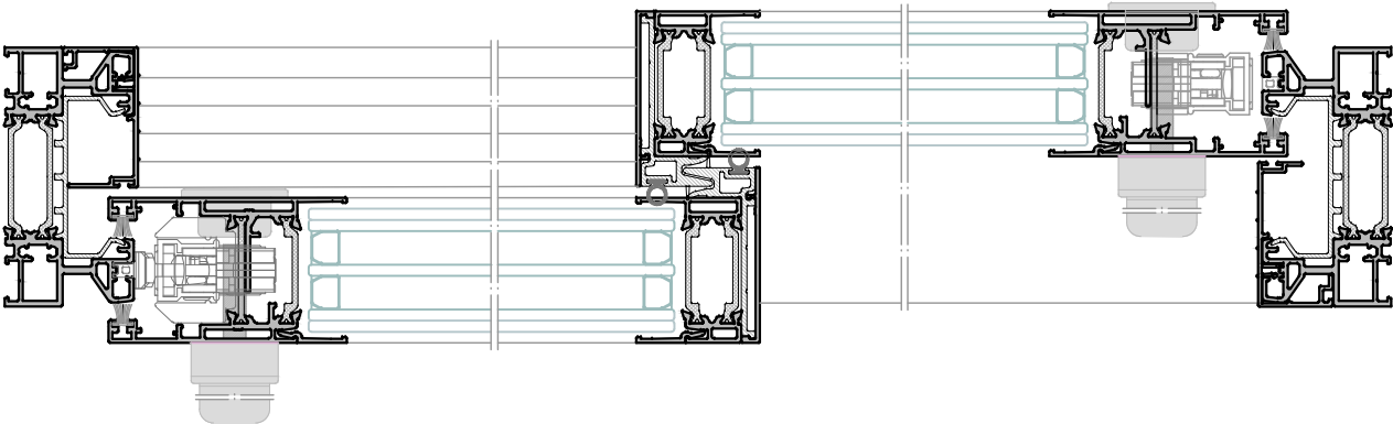
Sección A-A'
