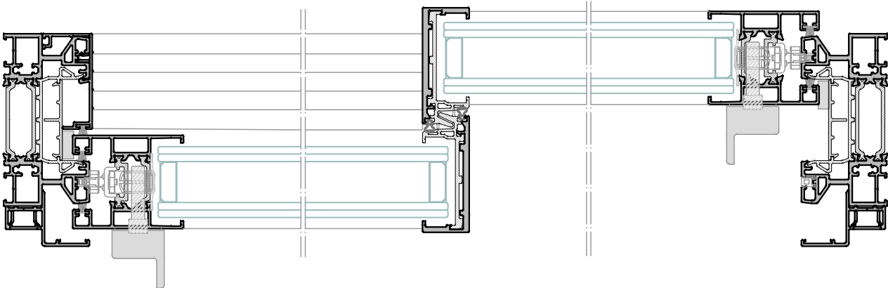
Sección A-A'
