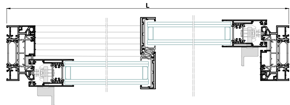
Sección A-A'
