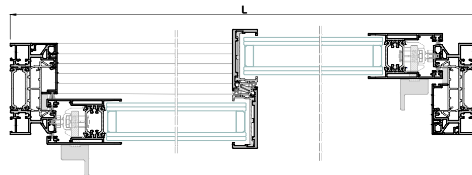
Sección A-A'
