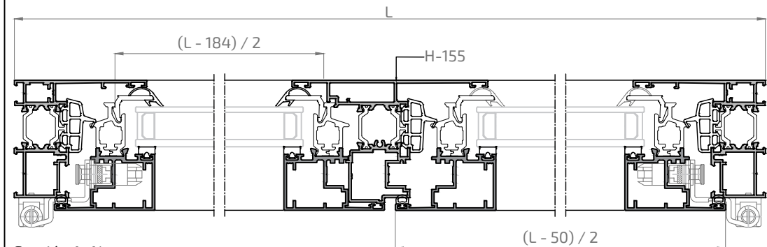
Sección A-A'
