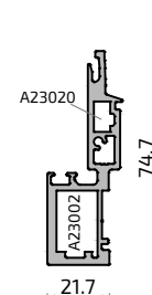
20844 Hoja Inver. Balconera ALG VISTA
