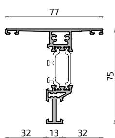
21309H Pilastra Reducida (junquillo de 32)
