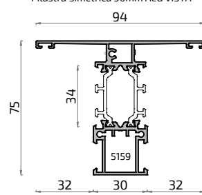
20941H Pilastra Simétrica 30mm ALG VISTA
