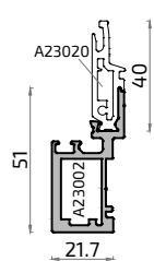
20713L Hoja Inversora ALG VISTA
