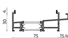
16319H NO STOCK Perfil Condensación
