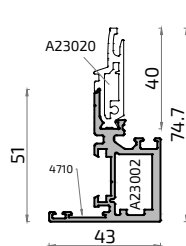
20712L Hoja ALG VISTA
