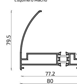
8592M Esquinero Macho
