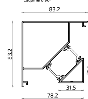
18215L Esquinero 90°
