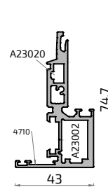
20845 Hoja Balconera ALG VISTA
