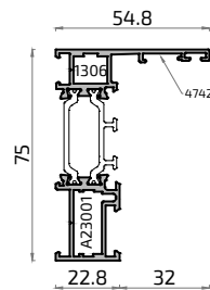
20705H Cercos ALG VISTA
