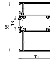
21541M Suplemento recogedor 65 mm
