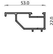
717 1207 Acople junquillo alg HS
