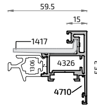
21428L Hoja Alg 65 Acríst. 43 mm
