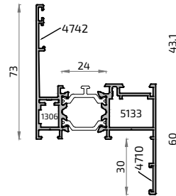
16768L Pilastra Simétrica 50 mm ALG 65 HS
