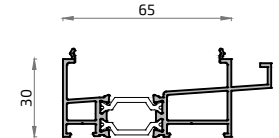
16319L NO STOCK Condensación 65 mm ALG 65
