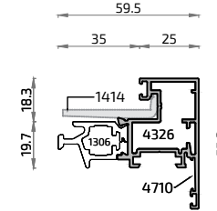
20223L Hoja Alg 65 HS
