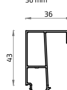
20218 Junquillo Largo 36 mm
