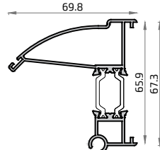
18897L Esquinero Regulable Hembra 65 mm
