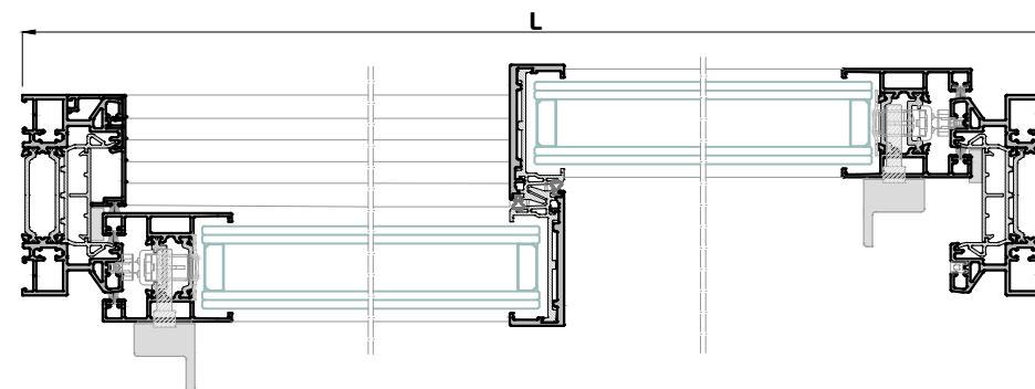
Sección A-A'
