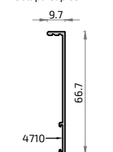
16323 Solapa Clip 65 mm
