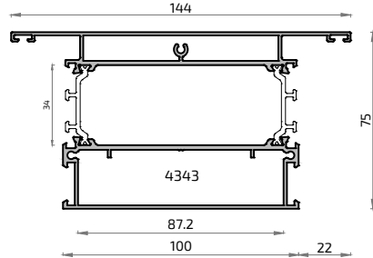
16310H Zócalo / Manguetón 100 ALG 75
