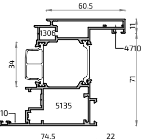
16336H Hoja Balconera ALG 75 C16
