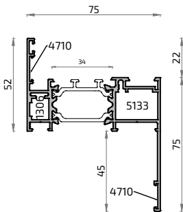
18181H Pilastra 60 mm ALG 75
