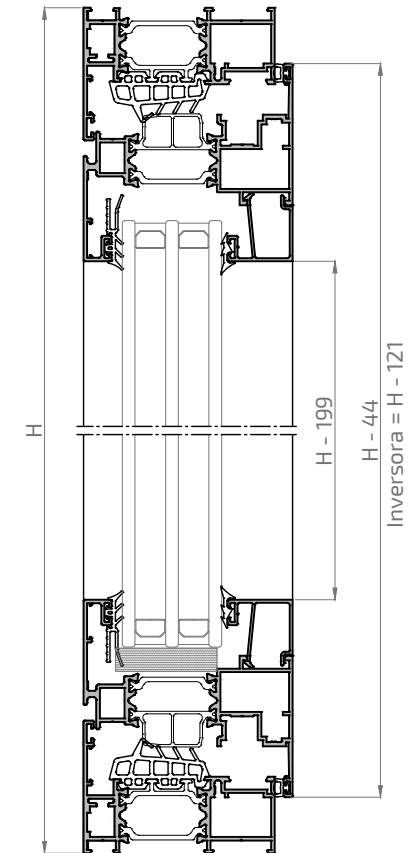
Sección B-B'
