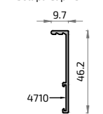
16322 Solapa Clip 45 mm
