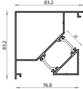
16322 Solapa Clip 45 mm
