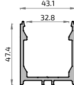
18420 Vierteaguas Inf. Cepillo
