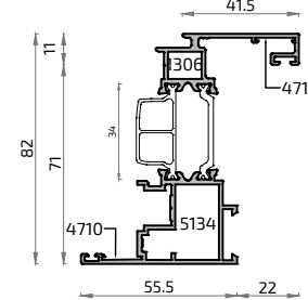
16334H Hoja Ventana ALG 75 C16
