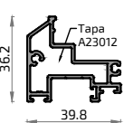
20338 Perfil Suelo Puerta
