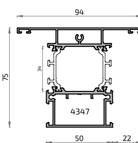
16310H Zócalo / Manguetón 100 ALG 75
