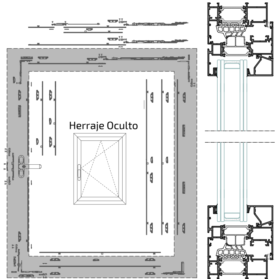
Sección B-B'
