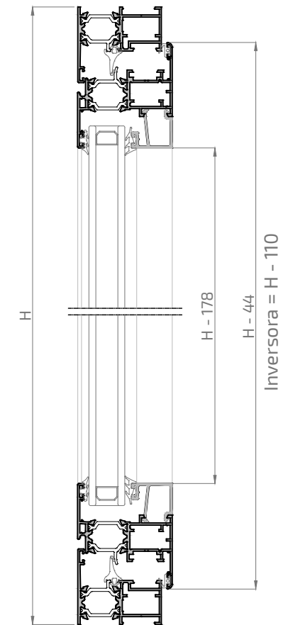
Sección B-B'
