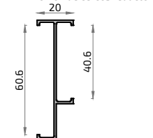
583 6653 Unión de cercos reductor
