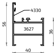
311 3586 Cercos Portada 36mm S-350E
