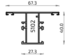
148 2593 Esquinero Regul. Tubo 40
