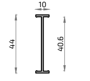
646 6144 Unión Cercos 40 mm
