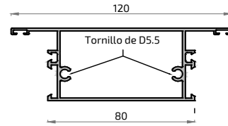
142 2579 Acople Vaivén S-100 y 350
