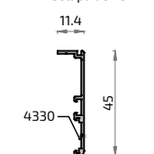
8629 Solapa de 45mm
