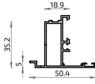
20140 Perfil Inversor
