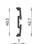
142 2579 Acople Vaivén S-100 y 350
