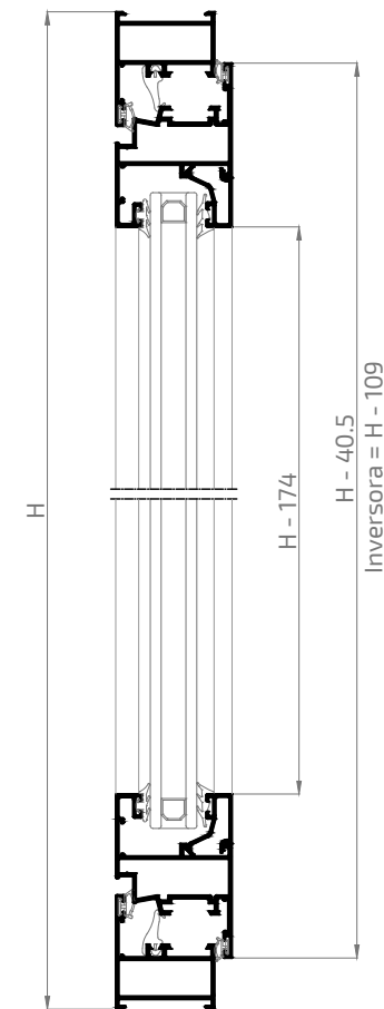
Sección B-B'
