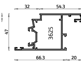
8296 Divisor Hoja s/junq. Dobl. Crist. S-350E
