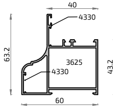
308 3583 Hoja Apertura Externa S-350E
