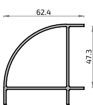
772 3592 Zócalo 100 mm S-350E
