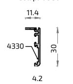
281 1140 Solapa de 30mm
