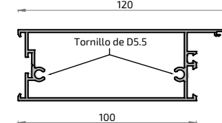
8629 Solapa de 45mm
