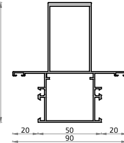
8891 Acople Manguetón Inf. Felpudo 4971
