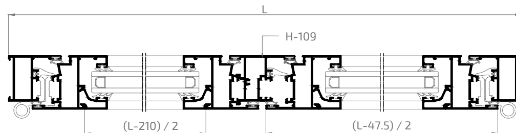
Sección A-A'
