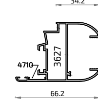
20143 Pilastra Reforzada Ancha
