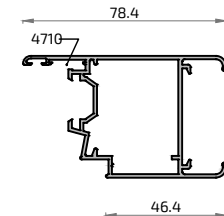
794 3603 Hoja Balconera S/Junq. S-350E
