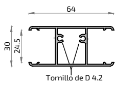
8296 Divisor Hoja s/junq. Dobl. Crist. S-350E
