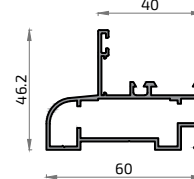
8593 NO STOCK Cercos Fijo Registro 60 mm S-350E
