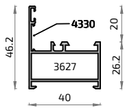
300 3575 Cercos de 40 mm S-350E
