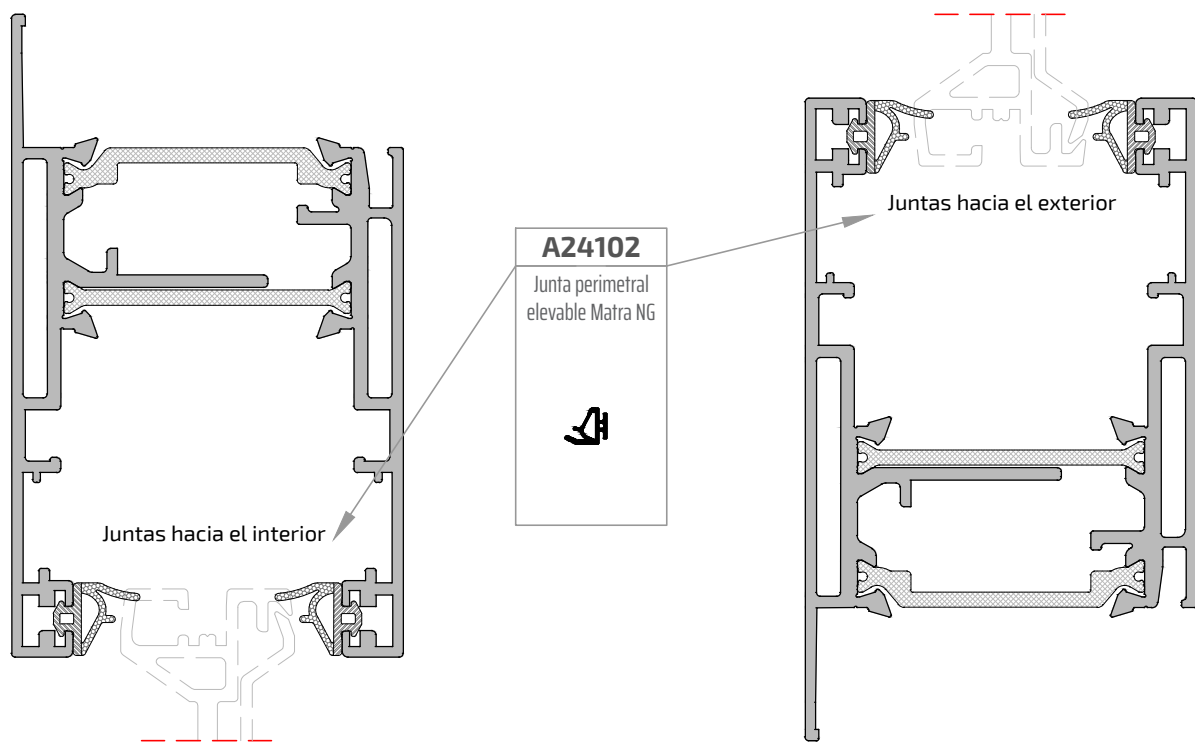
Posición de colocación de junta A24102 en perfiles inferior horizontal y laterales vertical.
