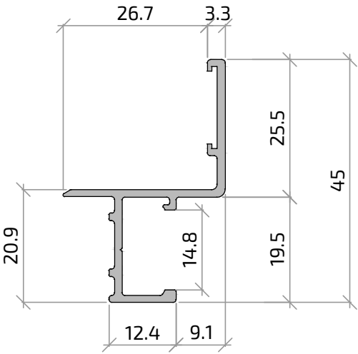
21251 Vierteaguas/Condensación
