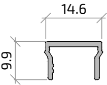
21209 Tapa clip
