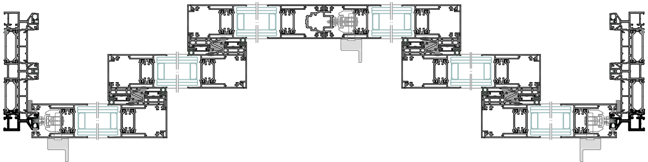
Sección 1-1'
