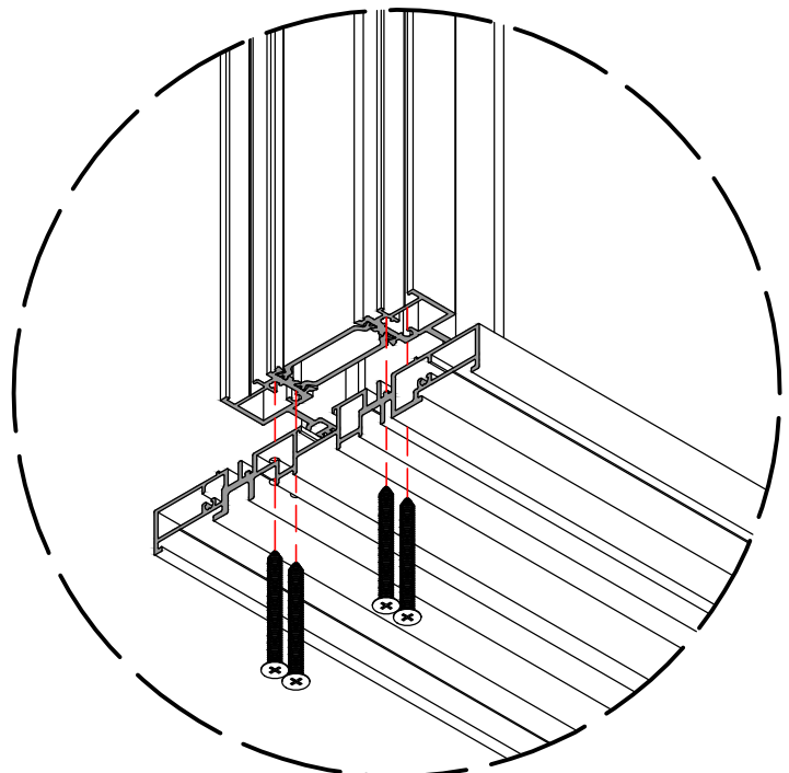
Detalle 3D cerco unión cerco empotrado
