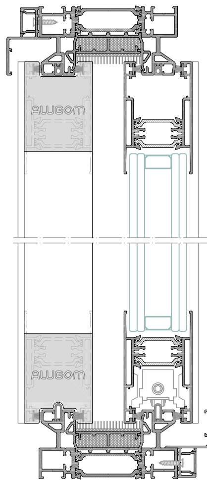
Sección 2-2'
