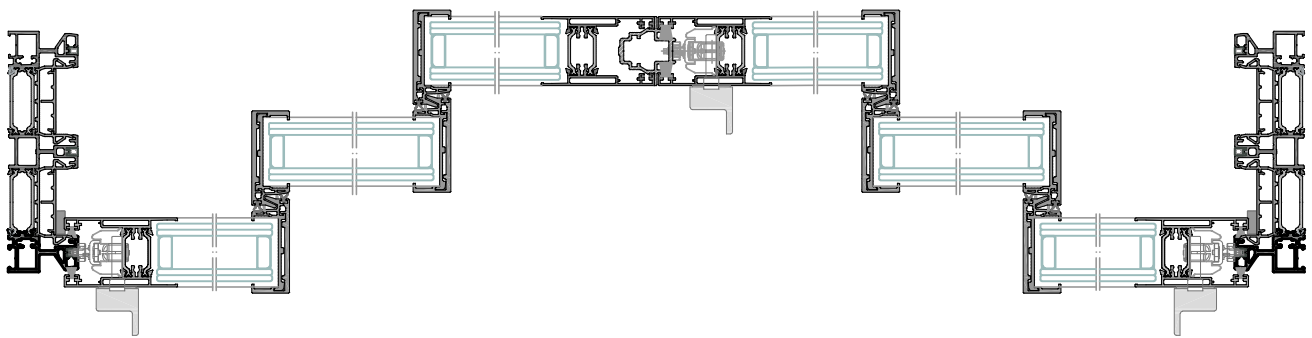
Sección 1-1'
