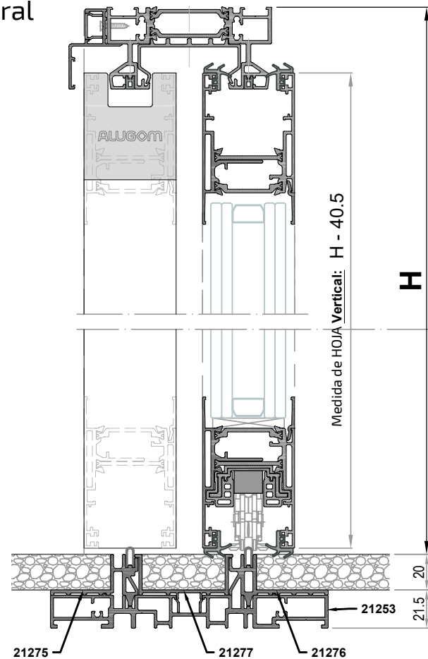
Sección B-B'
