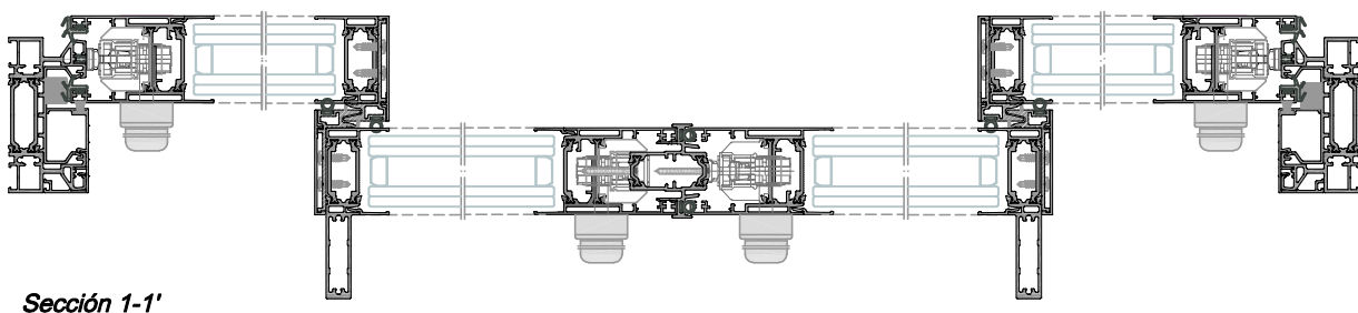
Sección 1-1'
