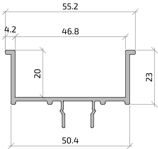
21277 Tapeta central cerco inf. empotrado
