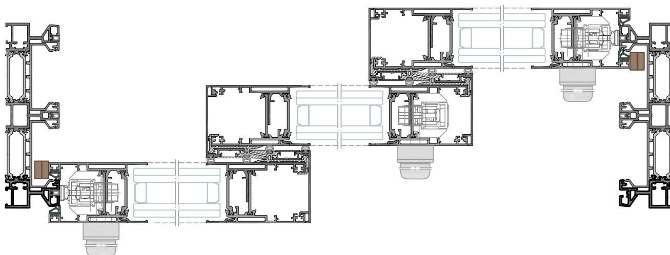
Sección 1-1'
