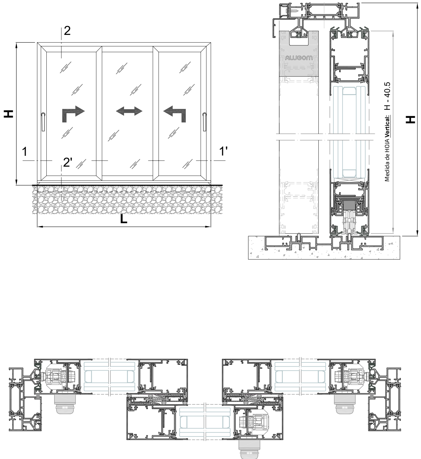
Sección 1-1'
