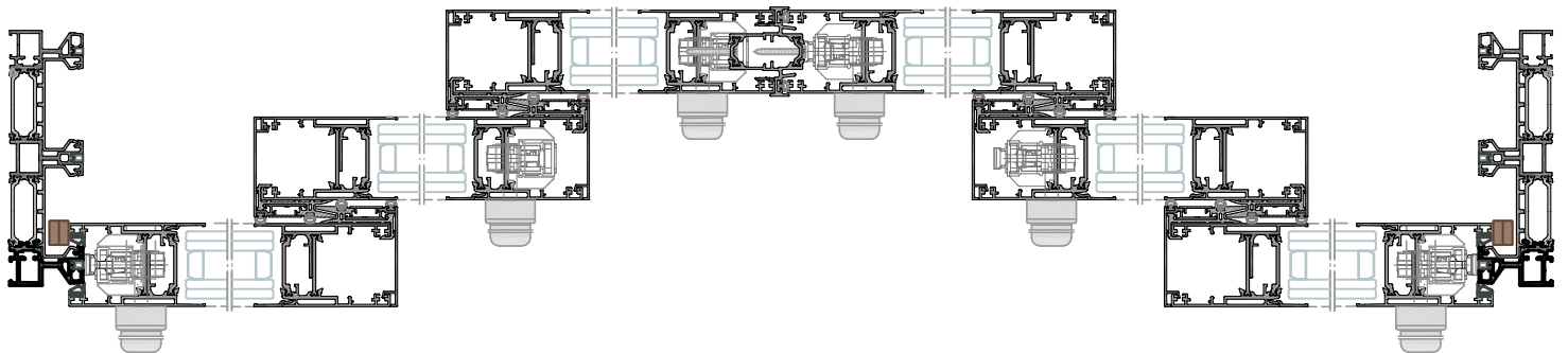
Sección 1-1'
