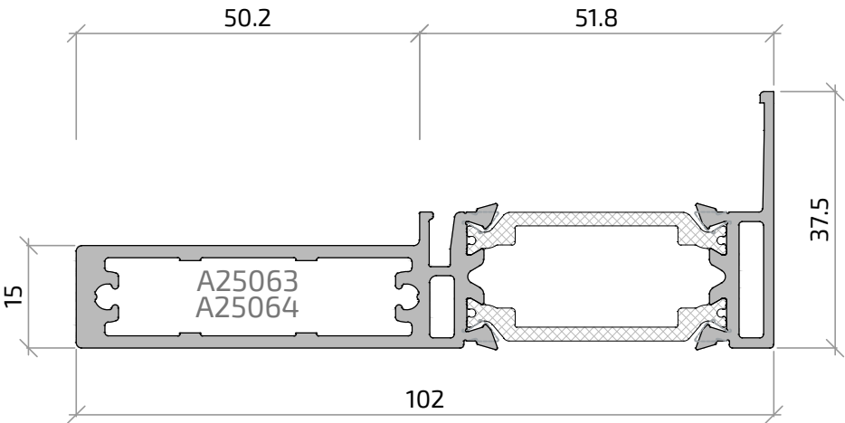
21274H Hoja central reforzada elevable interior
