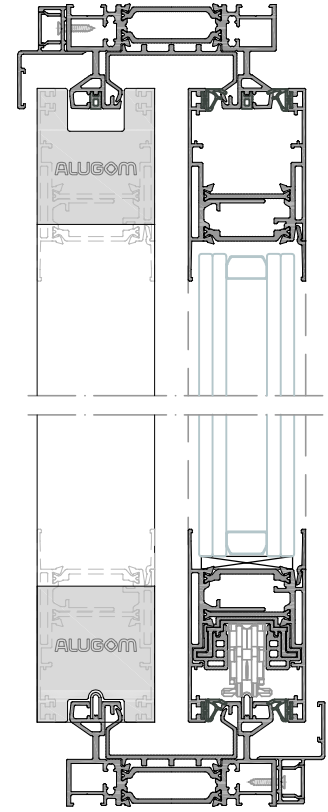
Sección B-B'
