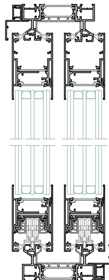
Sección B-B'
