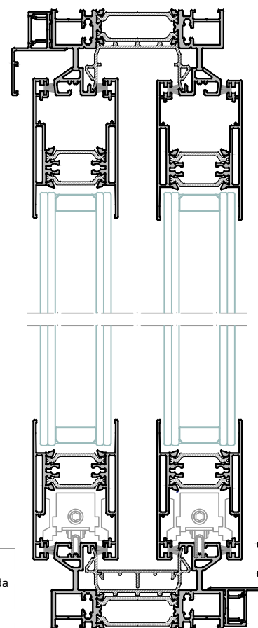
Sección B-B'
