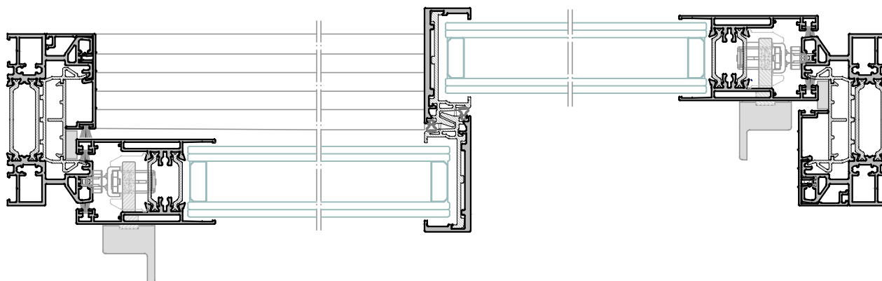
Sección A-A'
