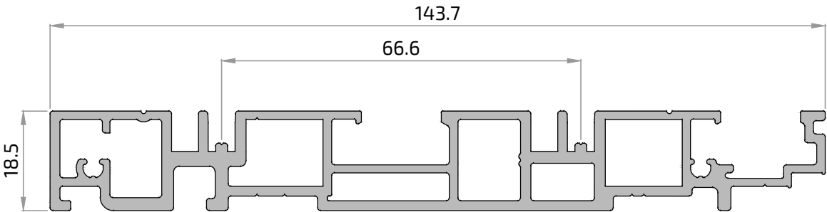
21699 Inicio Cerco multicarril Matra NG COVER*
