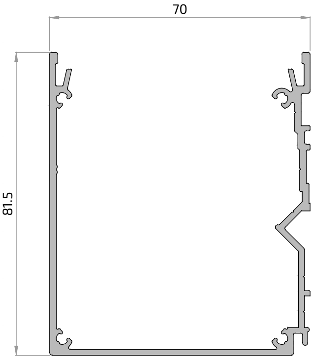
21691 Canalón Matra NG LINE
