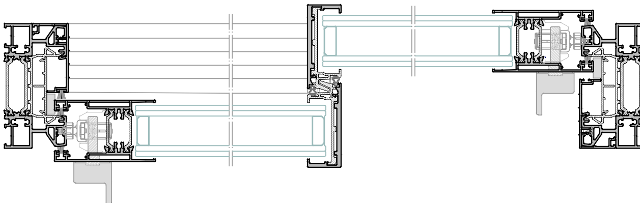
Sección A-A'
