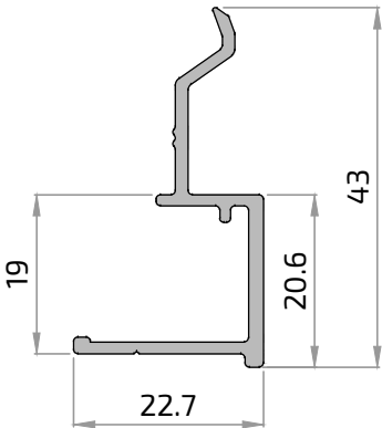
21678 Final Cerco multicarril Matra NG
