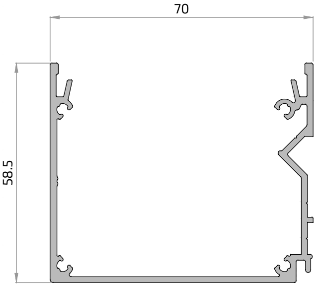
21690 Canalón Matra NG COVER
