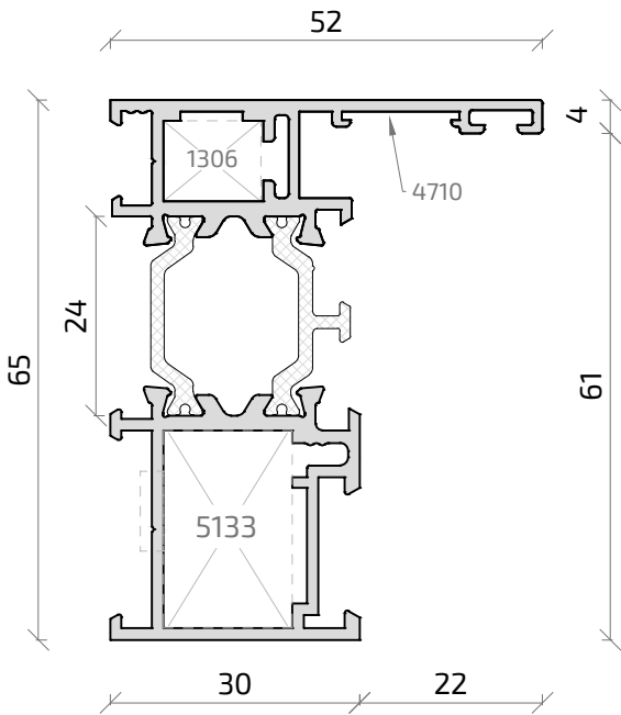
16332L Cerco 30 mm Alg 65
