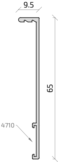
16323 Solapa Clip 65 mm
