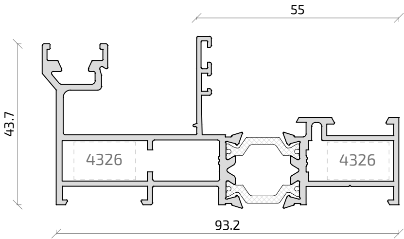
20195L Cerco Hoja-Fijo
