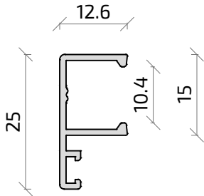
18272 Vierteaguas Postizo Alg Slide
