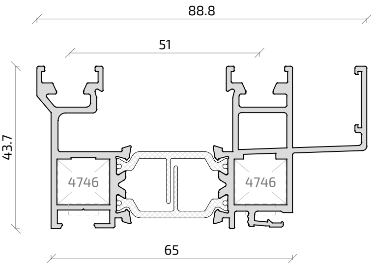
18146L Cerco 2C Alg Slide 65 Condensación grapa+clip
