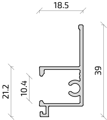
18135 Vierteaguas Alg Slide
