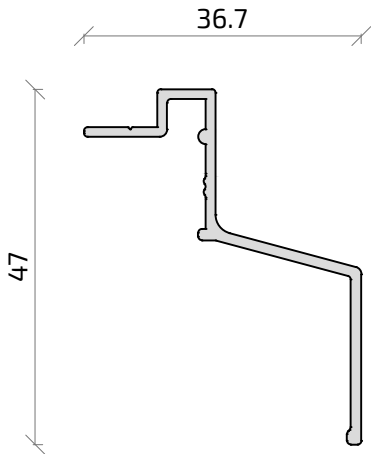
18873 Vierteaguas Alg Slide
