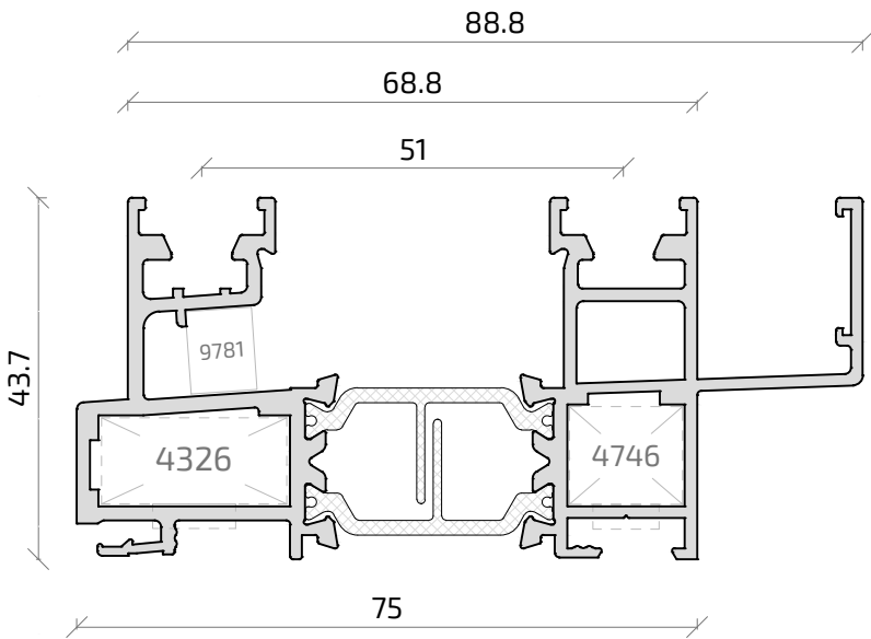
18144L NO STOCK Cerco 2C Alg Slide 75 Condensación clip+grapa
