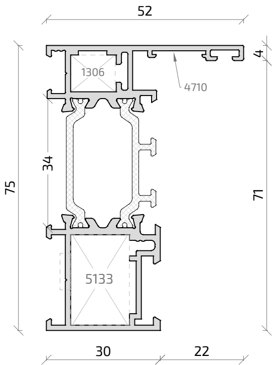
16332H Cerco 30 mm Alg 75
