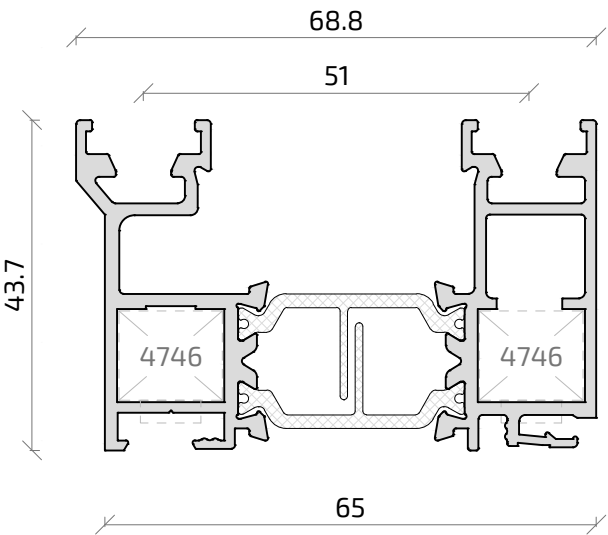
18145L Cerco 2C Alg Slide 65 grapa+clip
