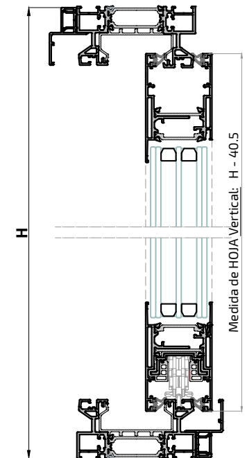
Sección B-B'
