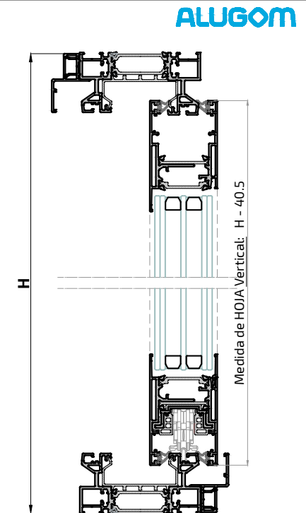
Sección B-B'
