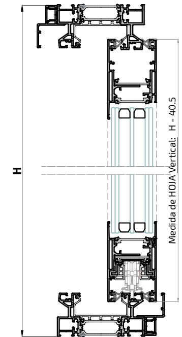
Sección B-B'
