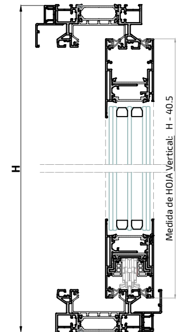
Sección B-B'
