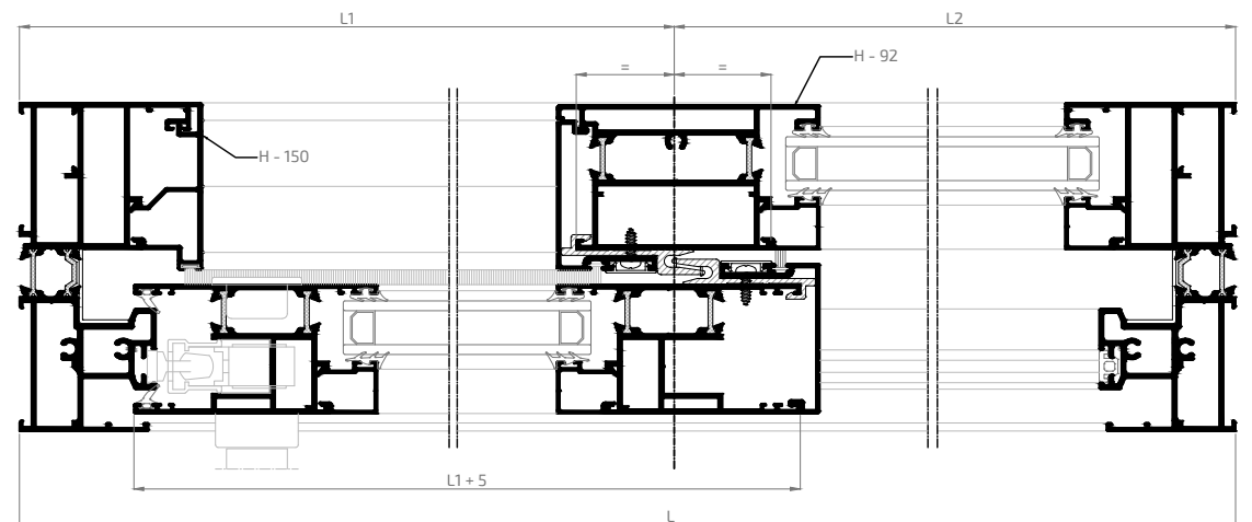
Sección A-A'
