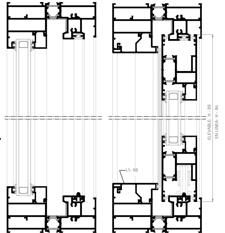
Sección C-C'
