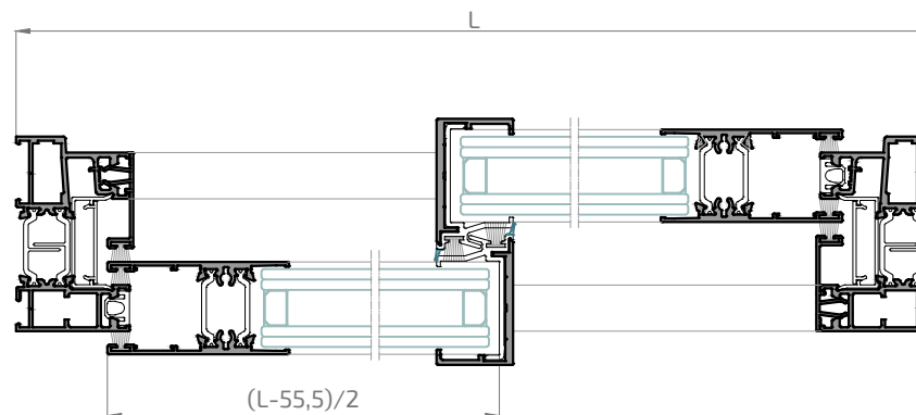
Sección A-A'
