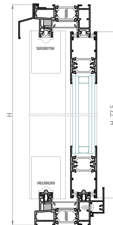
Sección B-B'
