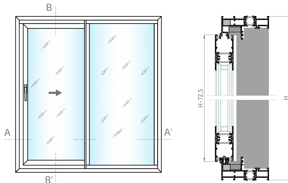
Sección B-B'
