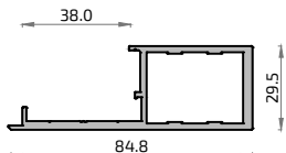
18145L Cercos 65 grapa+clip
