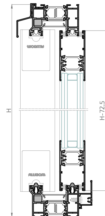
Sección B-B'
