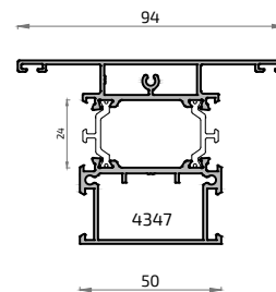
629 6807 Tapa Refuerzo Postizo
