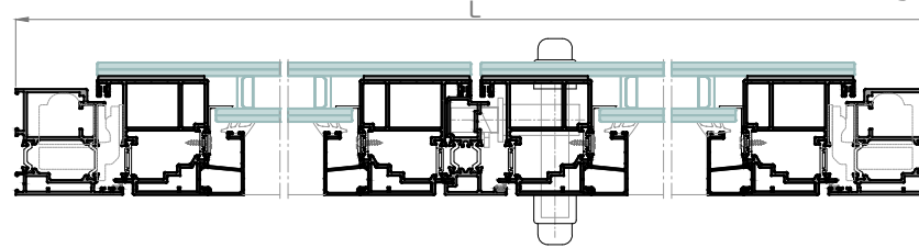
SECCIÓN A-A'
