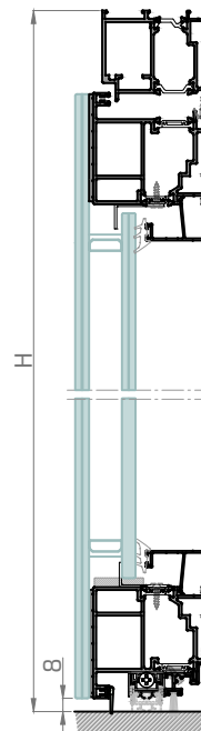
SECCIÓN B-B'
