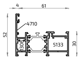
16332L Cercos 30 mm
