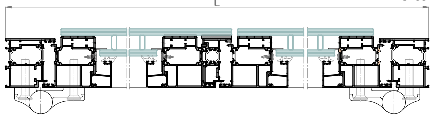
SECCIÓN A-A'
