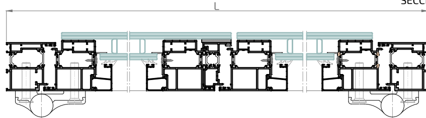
SECCIÓN A-A'
