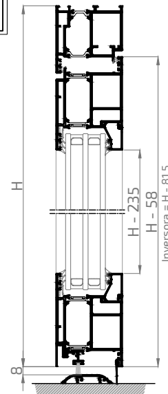
SECCIÓN B-B'
