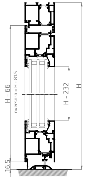
SECCIÓN B-B'
