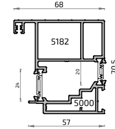
18152L Hoja Apertura Externa ALG GLASS
