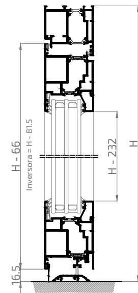
SECCIÓN B-B'
