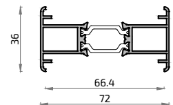
8482L Unión de Cercos 65 mm
