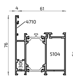
16300L Cerro 54 mm
