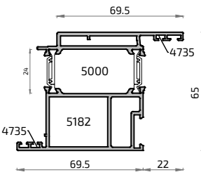
17187L Hoja ALG PUERTA Apert. Interna
