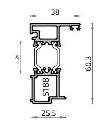
17279L Acople Inversora ALG PUERTA
