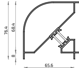
10006M Esquinero Curvo
