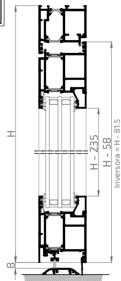
SECCIÓN B-B'
