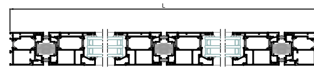
SECCIÓN A-A'
