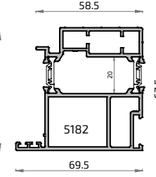
18271L Hoja apertura interna ALG GLASS
