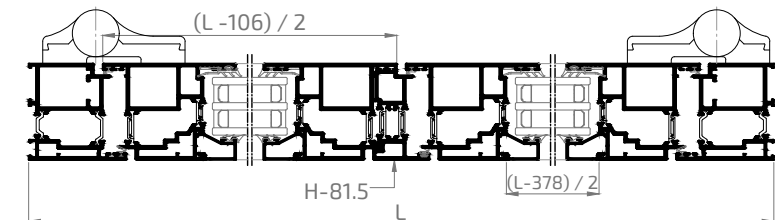
SECCIÓN A-A'
