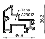
20338 Perfil Suelo Puerta
