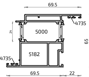
17187L Hoja ALG PUERTA Apert. Interna
