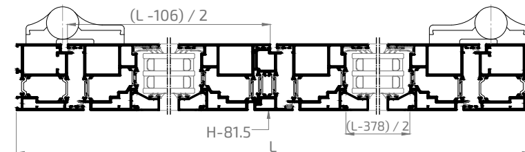
SECCIÓN A-A'
