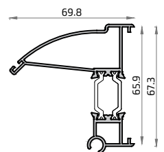
18897L Esquinero Regulable Hembra ALG 65
