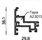
20355 Perfil Suelo Puerta
