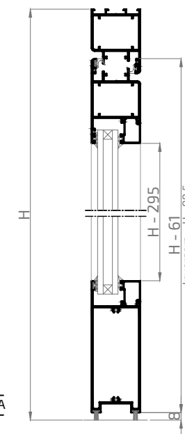
SECCIÓN B-B'
