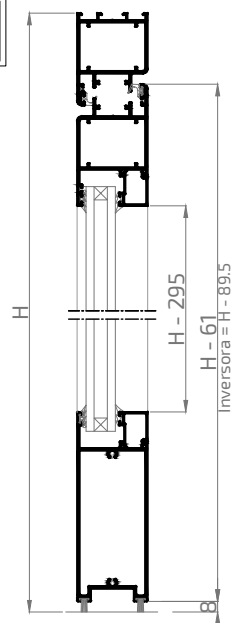
SECCIÓN B-B'
