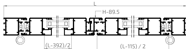
SECCIÓN A-A'
