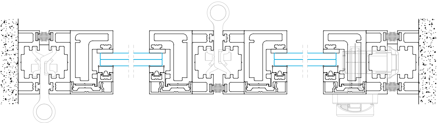
Sección A-A'
