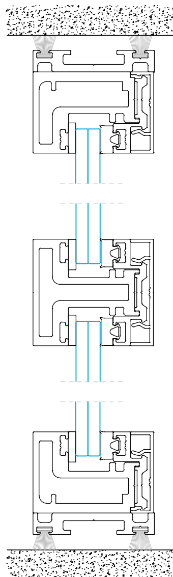
Sección B-B'
