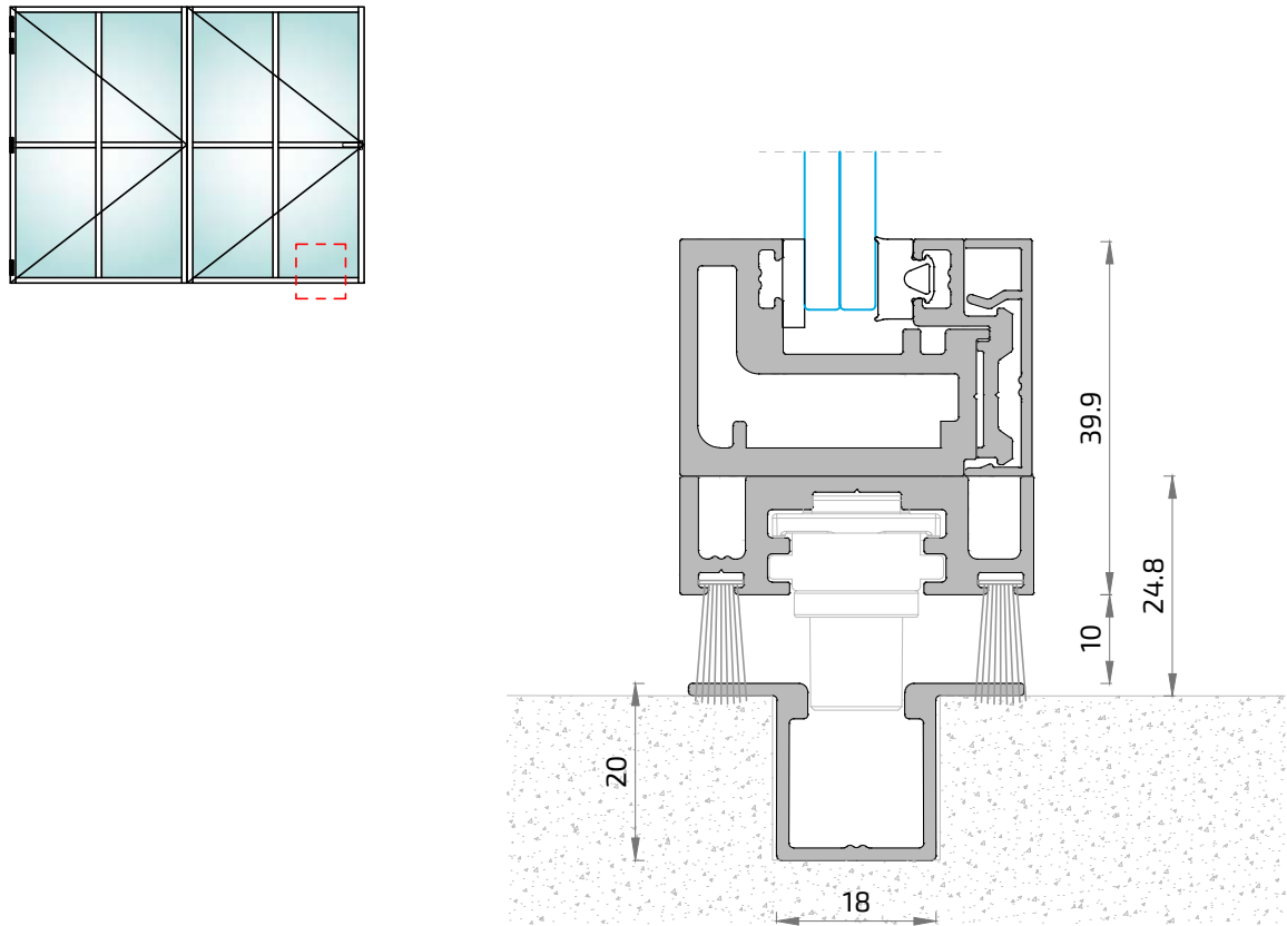
SECCIÓN Inferior Replegable hoja par
