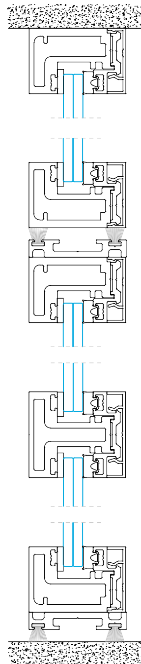
Sección B-B'
