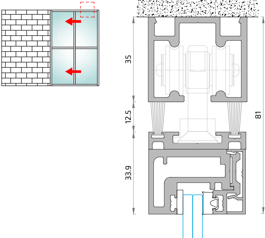
SECCIÓN Superior Corredera
