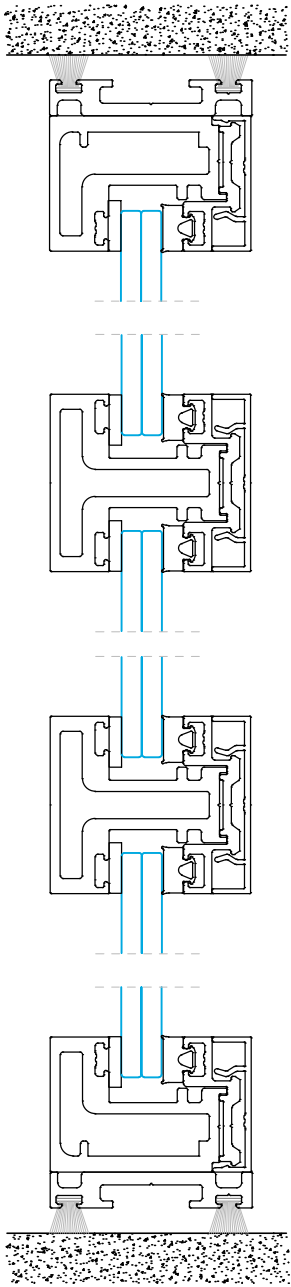
Sección B-B'
