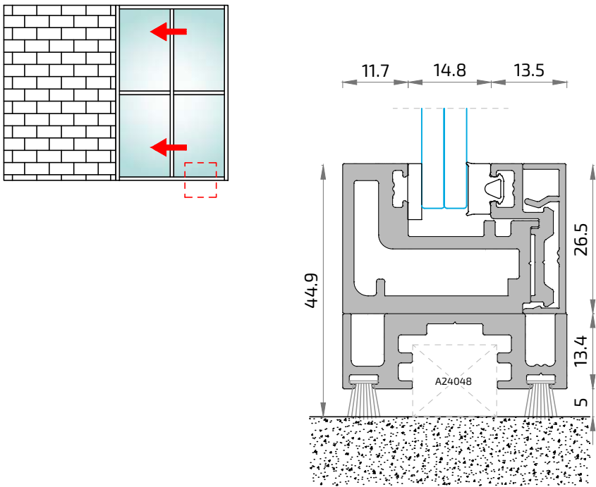
SECCIÓN Inferior Corredera
