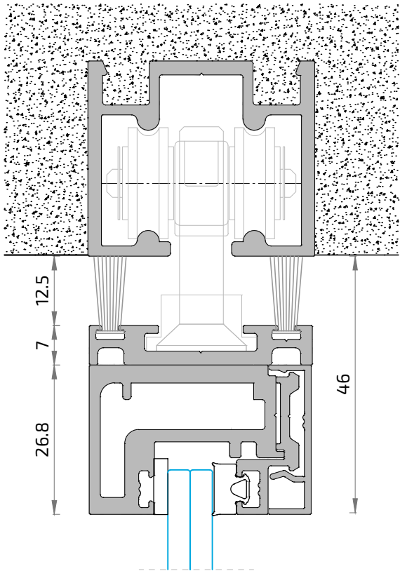
SECCIÓN Superior Corredera con guía encastrada
