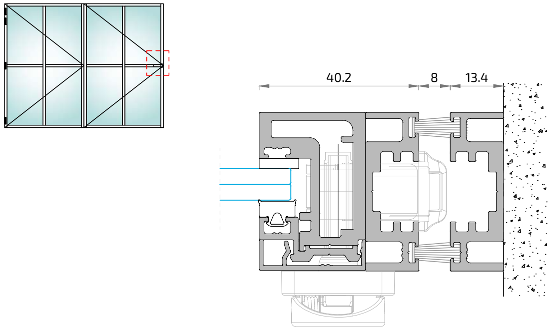
SECCIÓN Lateral Replegable con cerradura de pletinas
