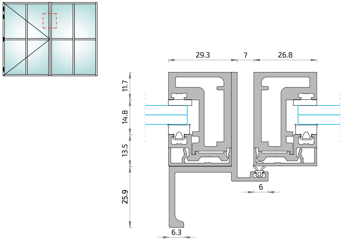
SECCIÓN Lateral Practicable con tirador batiente con fijo lateral
