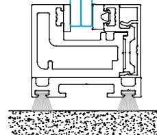
Sección C-C'
