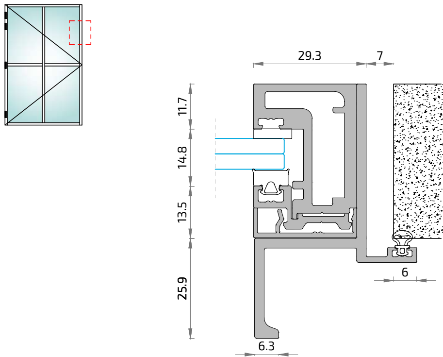
SECCIÓN Lateral Practicable con tirador con batiente
