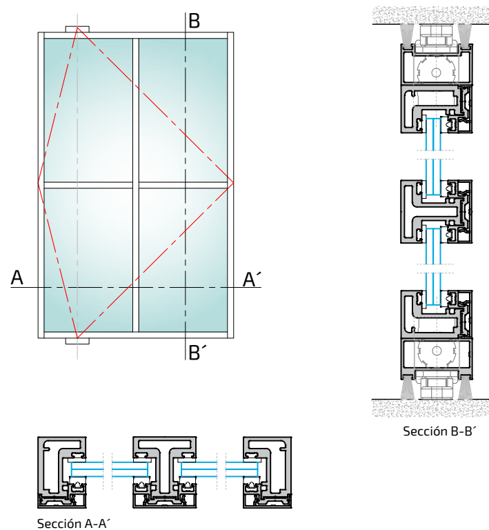
Sección A-A'
