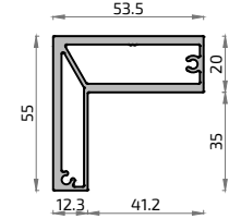
21121 Perfil Soporte Guía Corredera para Pared NOVA
