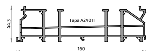
20994 Premarco Desagüe 160
