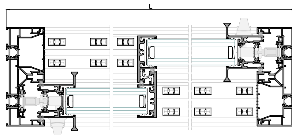
Sección A-A'
