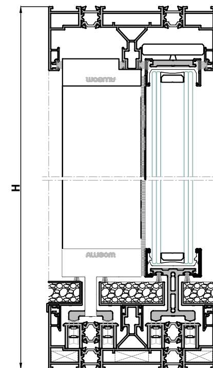
Sección B-B'
