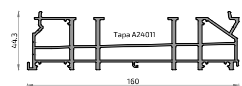
20994 Premarco Desagüe 160
