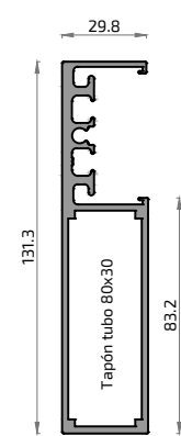
20993 Premarco Desagüe 80
