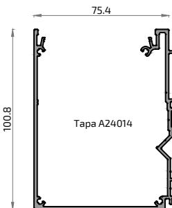
20978 Canalón 100 I-Cover
