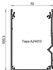
20979 Canalón 100 Ibiza
