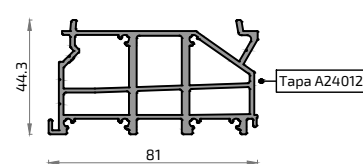
20993 Premarco Desagüe 80
