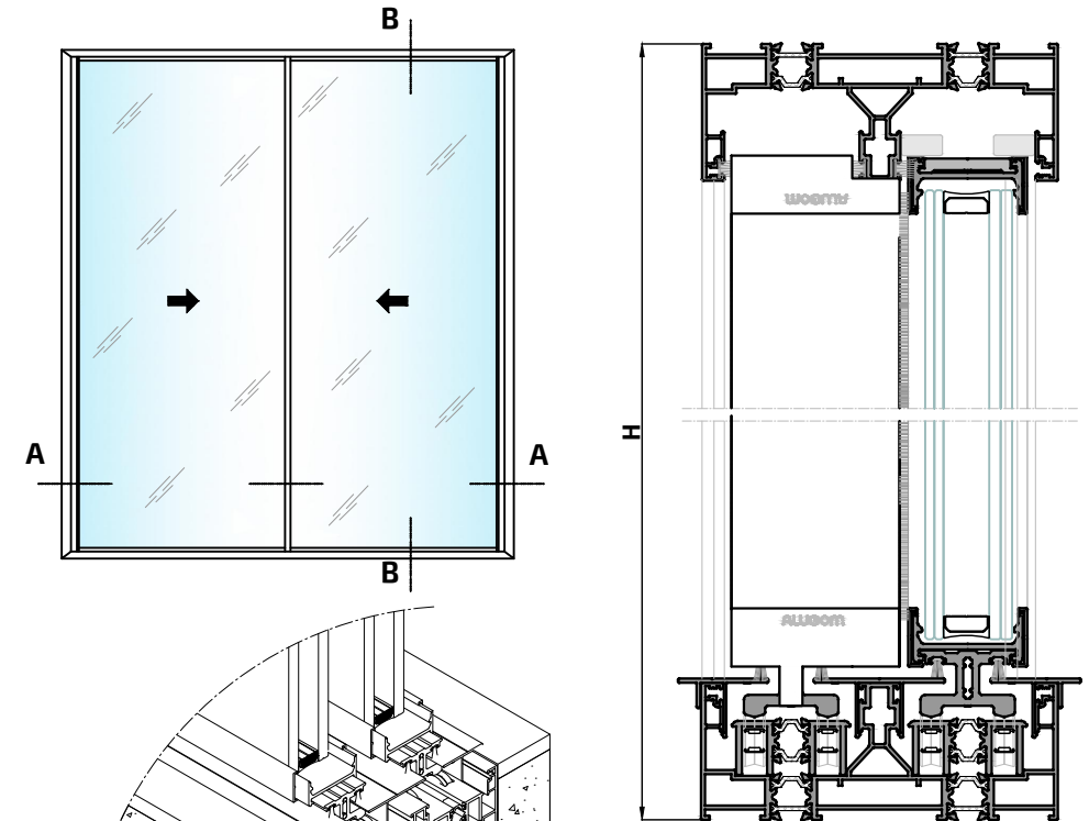
Sección B-B'
