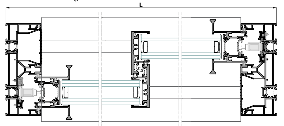
Sección A-A'
