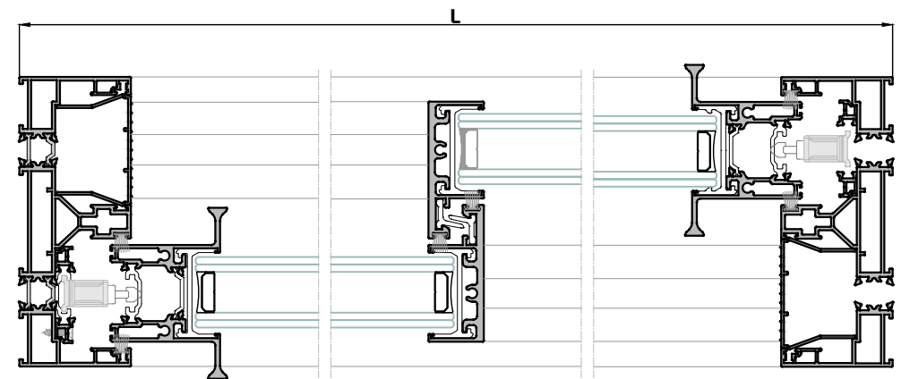
Sección A-A'
