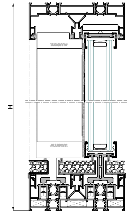
Sección B-B'
