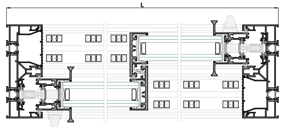
Sección A-A'
