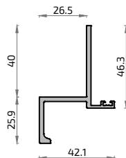
21209 Tapa Clip
