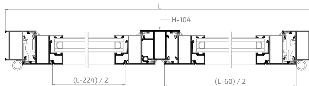
Sección A-A'
