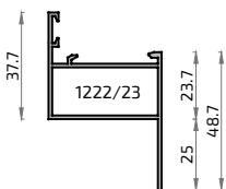
134 2542 Cercos con Solapa S-100
