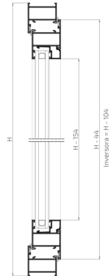
Sección B-B'
