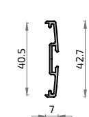
142 2579 Acople Vaivén S-100 y 350
