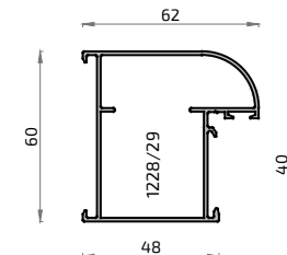
180 2591 Cercos Escaparate 48 mm S-100
