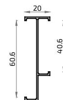
583 6653 Unión de cercos reductor
