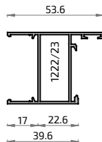
138 2534 Hoja para Lamas S-100
