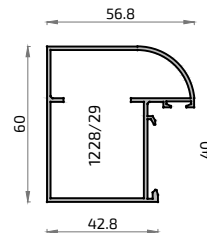
126 2526 Cercos Escaparate 43 mm S-100
