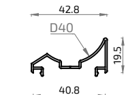
148 2593 Esquinero Regul. Tubo 40
