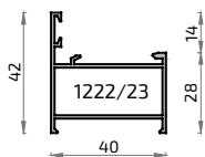
100 2541 Cercos 28 mm S-100
