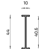
646 6144 Unión cercos 40 mm
