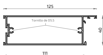
123 2507 Cercos Zócalo 111 mm S-100
