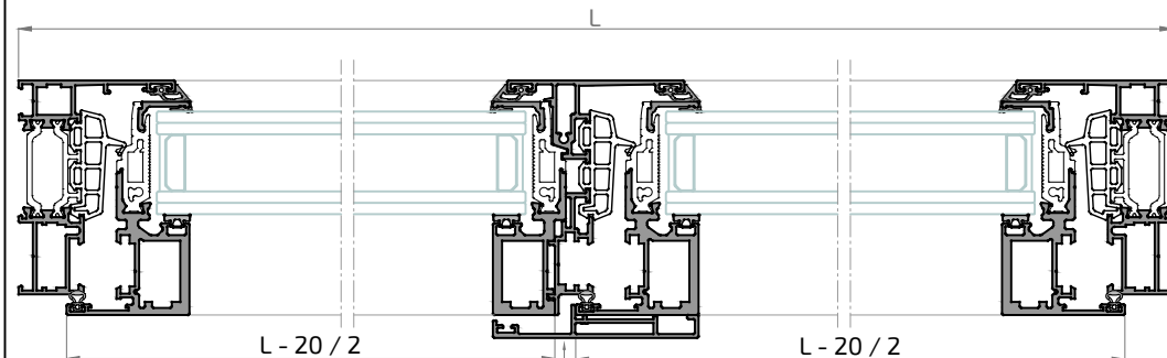
Sección A-A'
