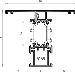
20941H Pilastra Simétrica 30mm ALG VISTA
