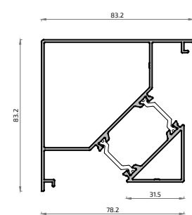
18215L Esquinero 90°
