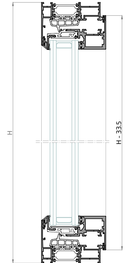
Sección B-B'
