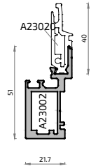
20713L Hoja Inversora ALG VISTA
