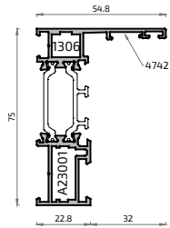
20705H Cercos ALG VISTA
