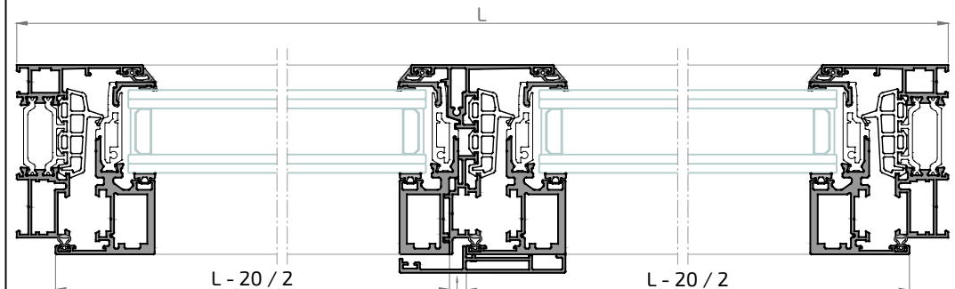
Sección A-A'
