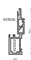
20844 Hoja Inver. Balconera ALG VISTA
