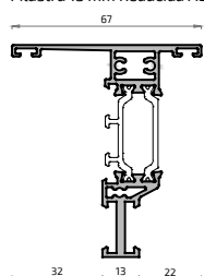
20840H Pilastra 13 mm Reducida ALG VISTA
