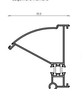
8591M Esquinero Hembra
