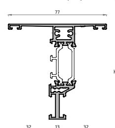
21309H Pilastra Reducida (junquillo de 32)
