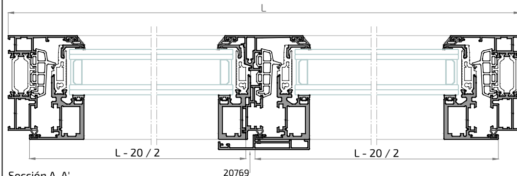
Sección A-A'
