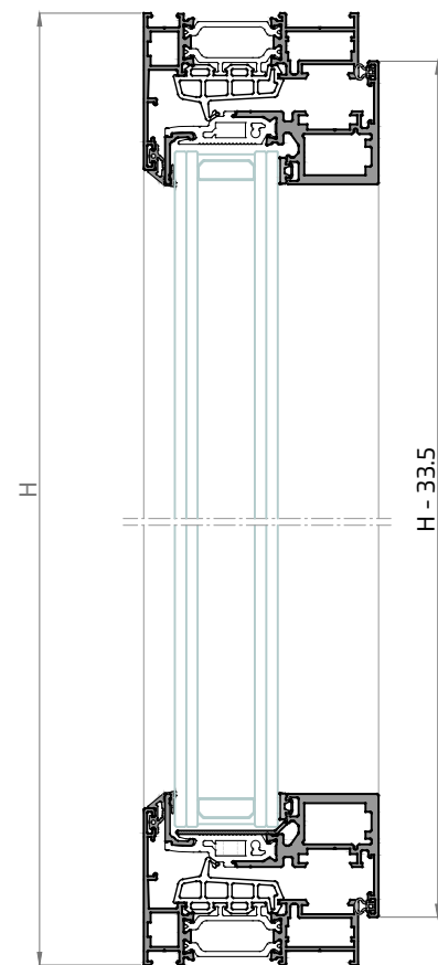
Sección B-B'
