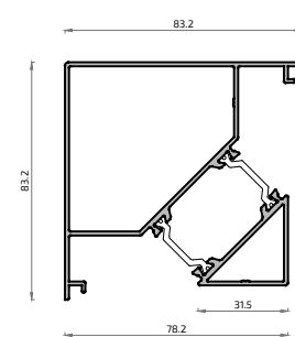
18215L Esquinero 90°
