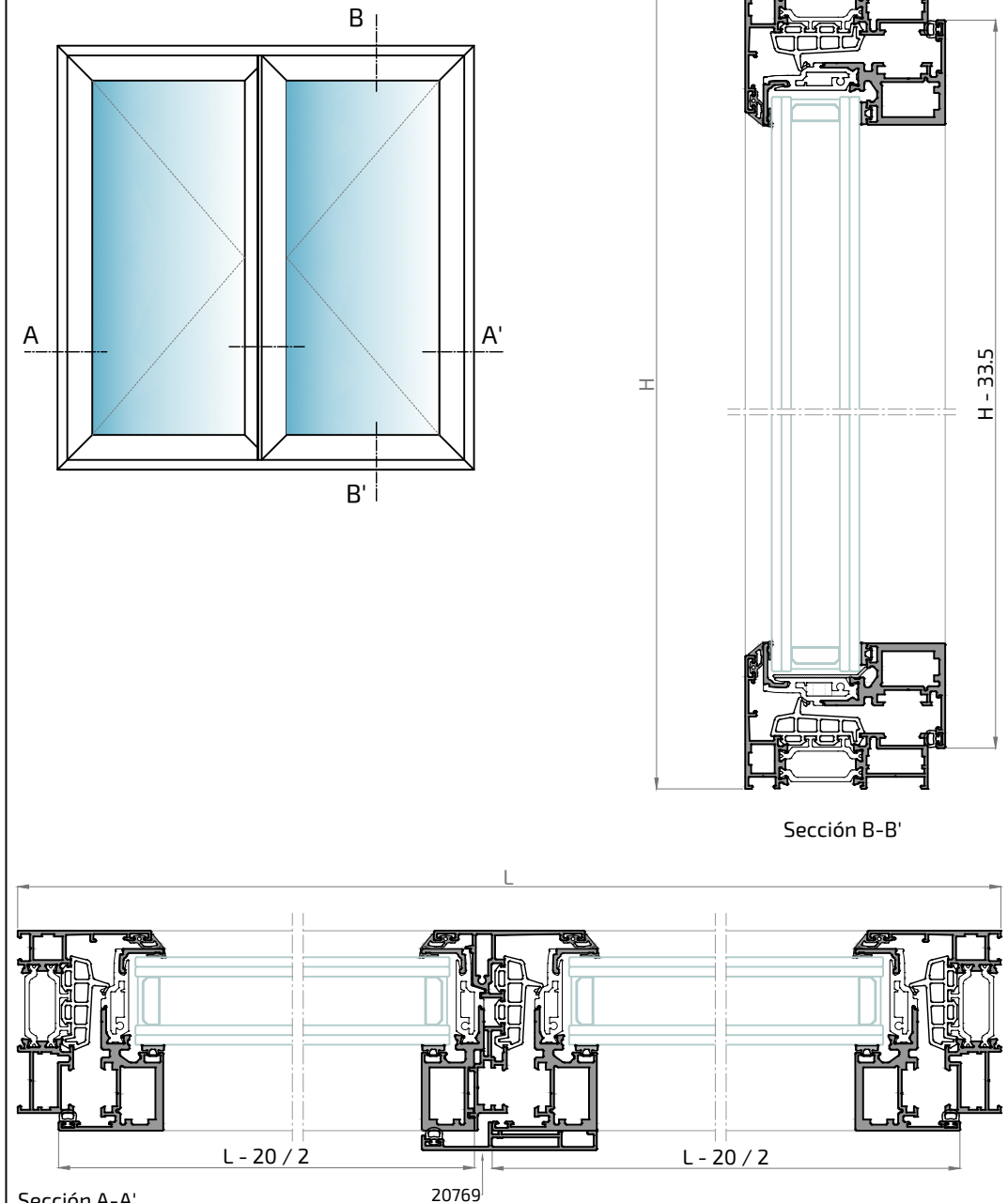
Sección A-A'
