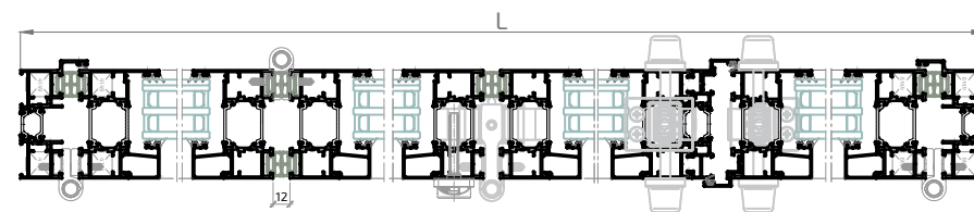
Sección A-A'
