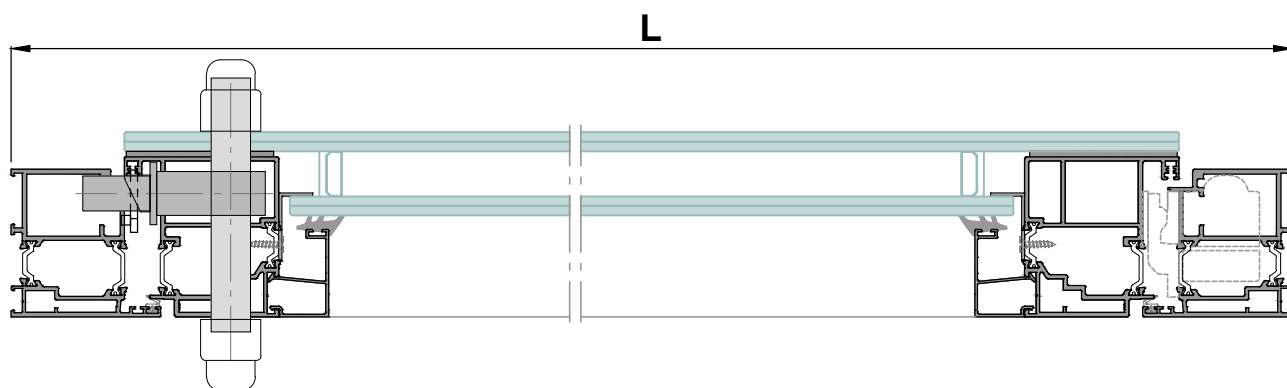
Sección A-A'
