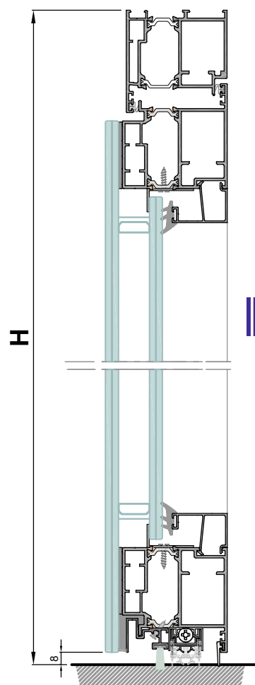
Sección B-B'
