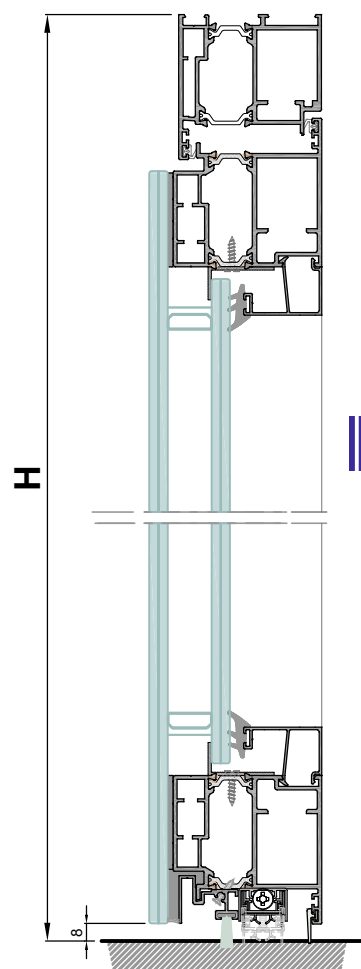
Sección B-B'
