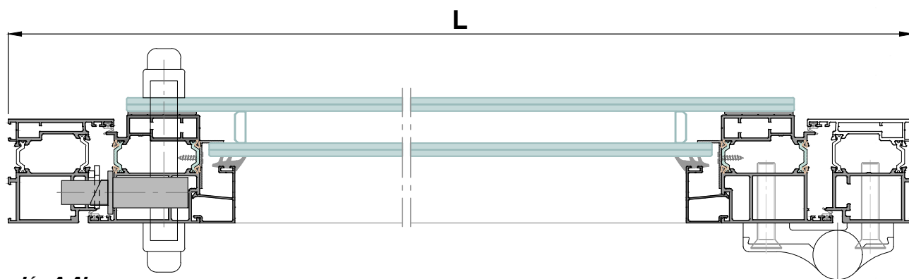
Sección A-A'
