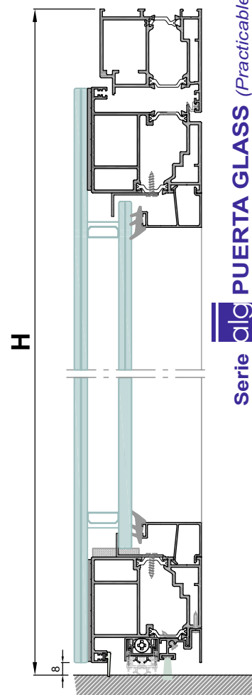
Sección B-B'
