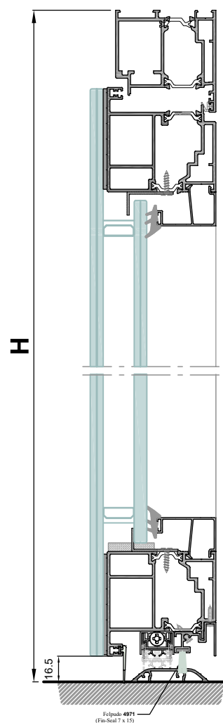
Sección B-B'
