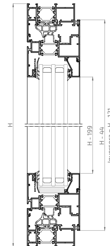
Sección B-B'
