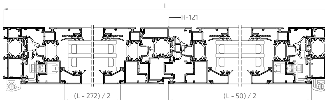
Sección A-A'
